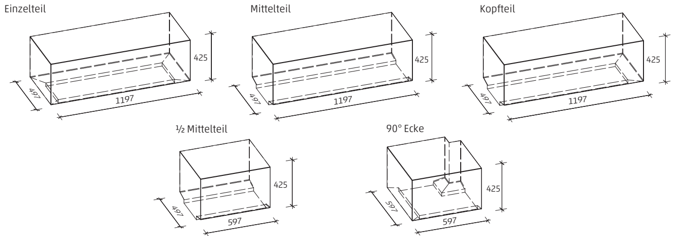
Holzauflagen Querlattung
