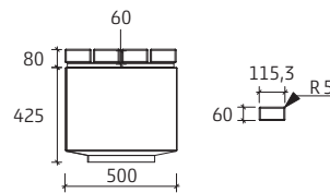
Holzauflagen Längslattung
