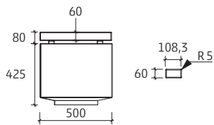
Holzauflagen Querlattung
