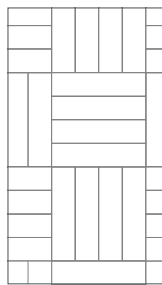
Parkett-Verband
