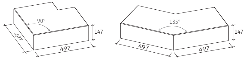
rinnit Eckblockstufen
