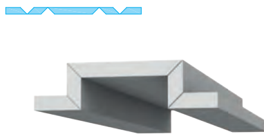
2 + 2 90° V-Fräsungen
