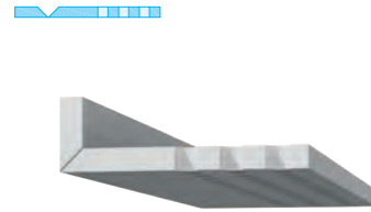
2x 90° V-Fräsungen
