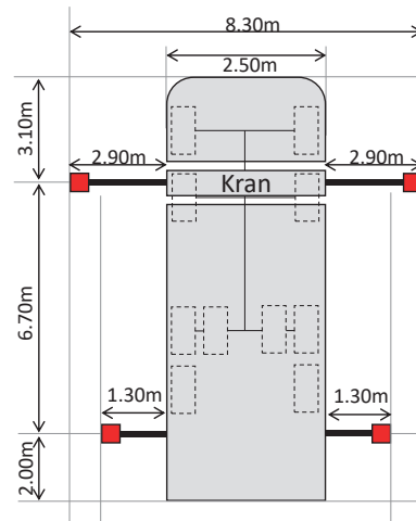
Lastwagen mit Kran 28 m
