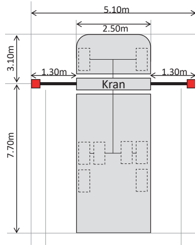
Lastwagen mit Kran 9 m
