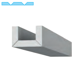
3x 90° V-Fräsungen
