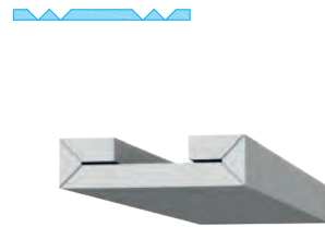
4x 90° V-Fräsungen + Plattenstreifen
