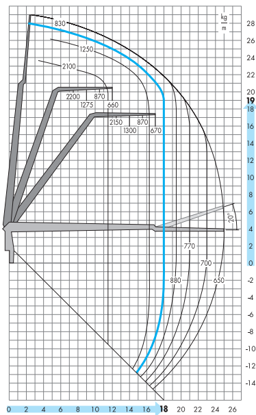
Lastwagen mit Kran 28 m
