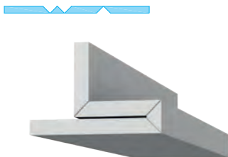
2 + 1 90° V-Fräsungen
