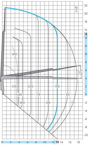
Lastwagen mit Kran 9 m
